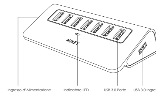
Ingresso d'Alimentazione Indicatore LED USB 3.0 Porte USB 3.0 Ingresso
